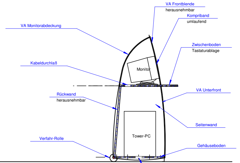
Schnitt
