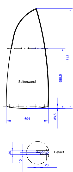
Vorderansicht
