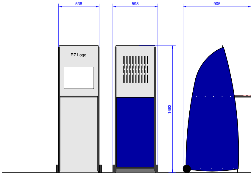
Vorderansicht
