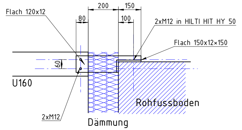
Detail Auflager/Befestigung 2mal
